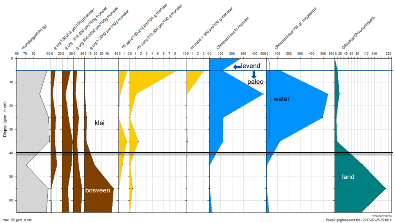
Figuur 2. Diagram van de fysische eigenschappen van de monsters en ecologische kengetallen.
