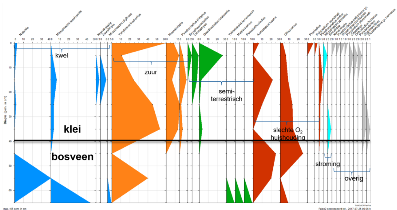
Figuur 3. Diagram van de Chironomidae, ingedeeld naar voornaamste eigenschap van de afzonderlijke soorten.
